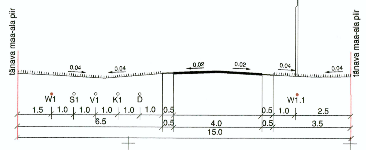
LÕIGE 1 - 1 M1:100
