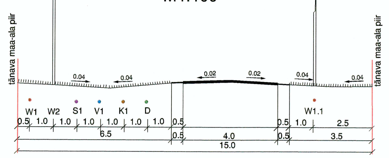
LÕIGE 1A - 1A M1:100
